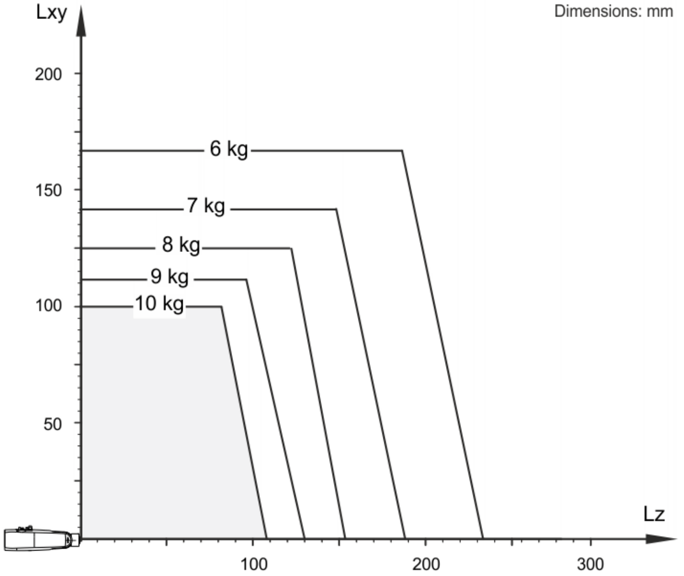
KR 10 R900 CR 负载能力图表
