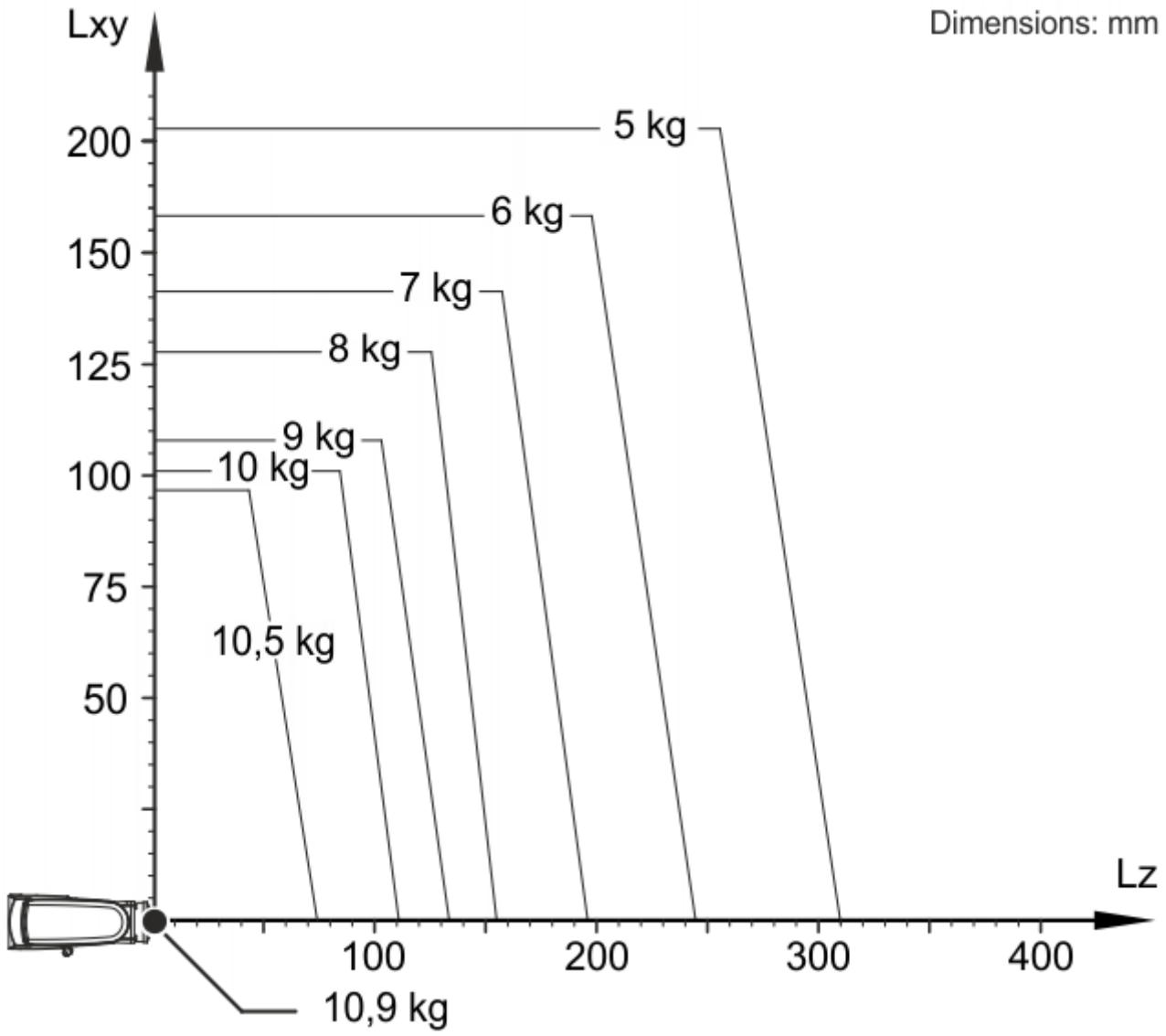
KR 10 R1100-2 负载能力图表
