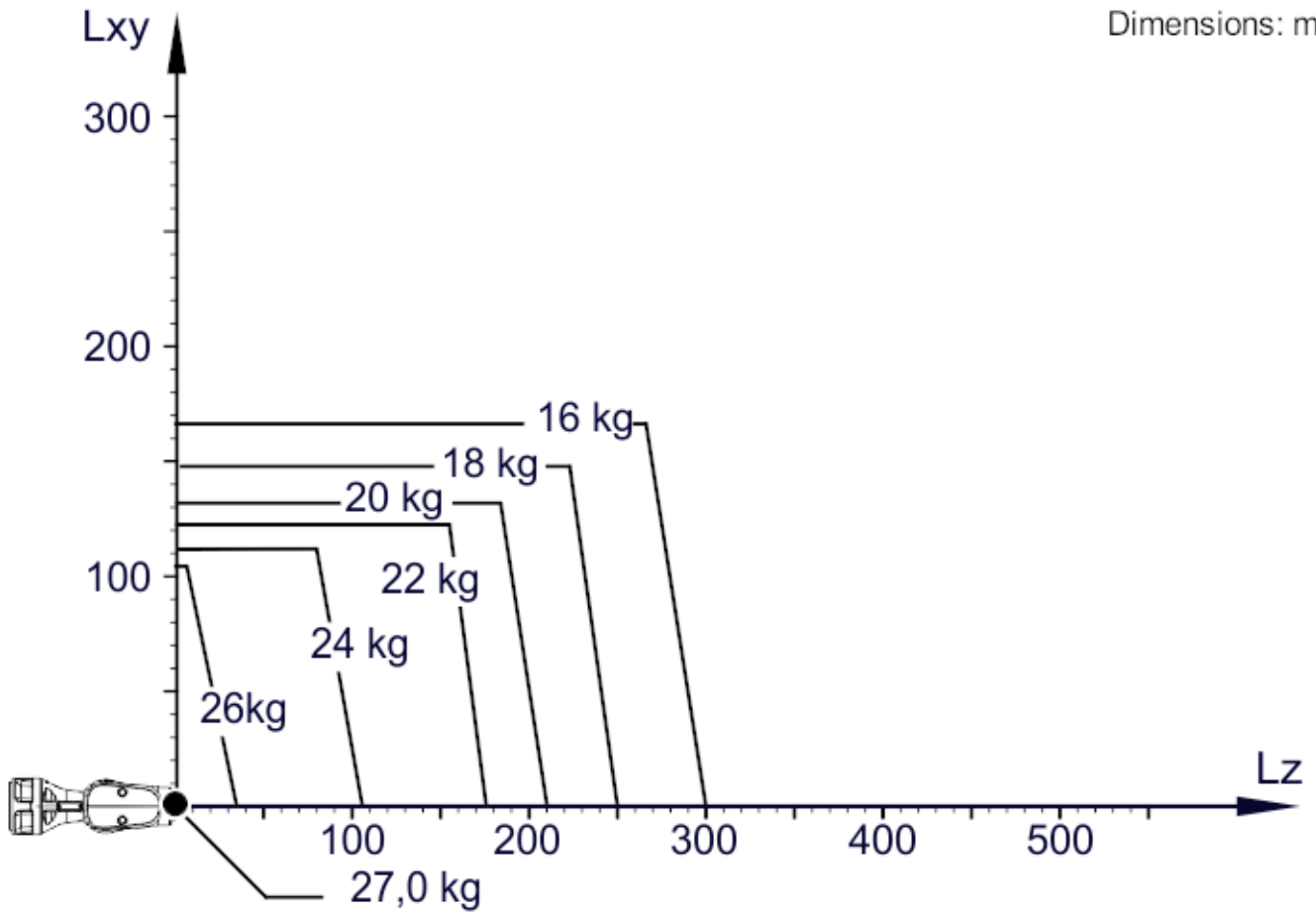
KR 22 R1610 负载能力图表
