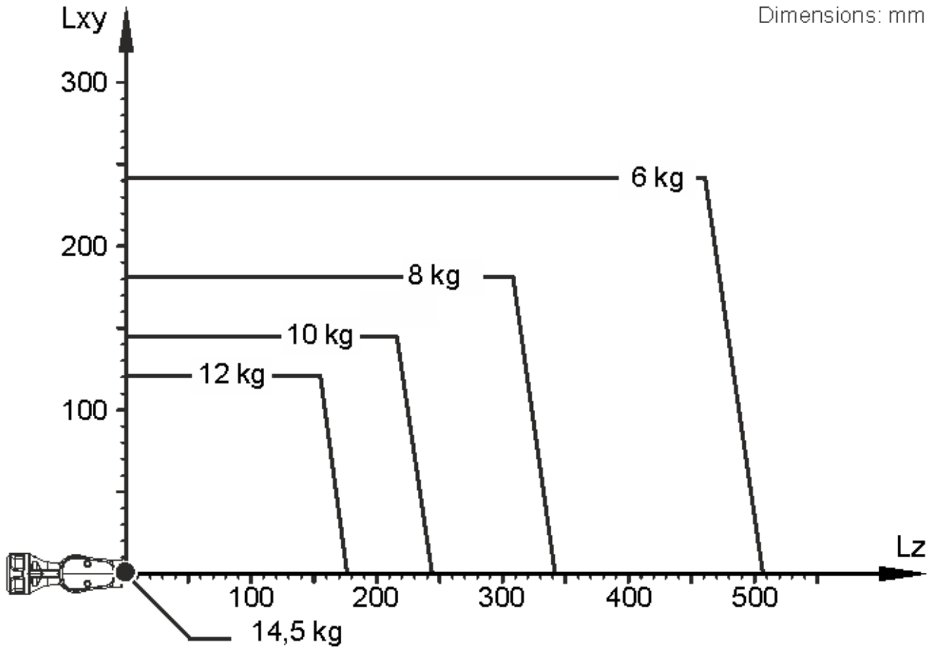
KR 12 R1810-2 负载能力图
