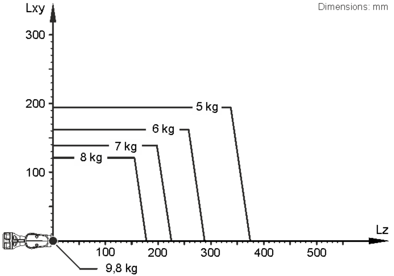
KR 8 R2010-2 负载能力图
